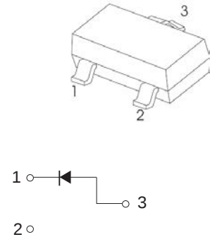
SOT-23
